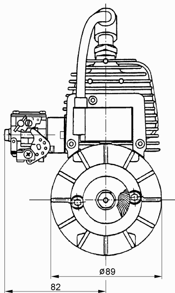
TITAN ZG 38SC Maßstab 1:3
